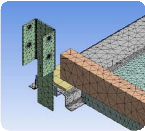
Modelo 3D de Perfil Omega Soporte. Mallado FEM.
