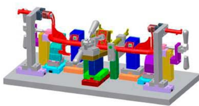
Diseño 3D Utillaje de Control
